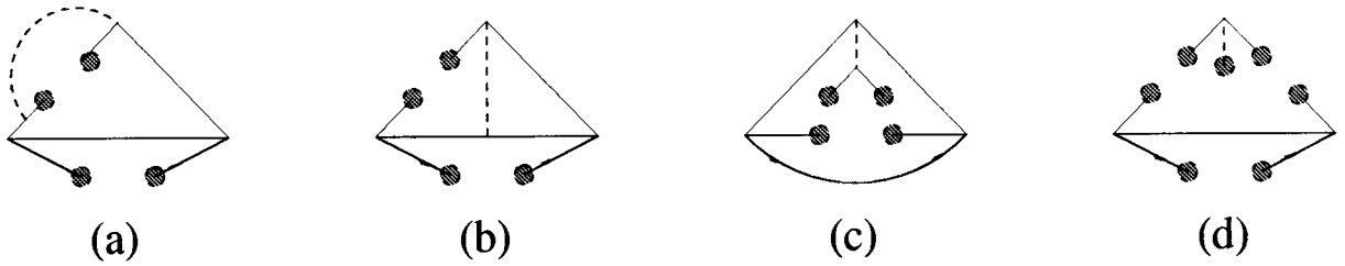
FIG. 3. Typical local (a,b,c) and bilocal (d) power corrections of dimension 6.
